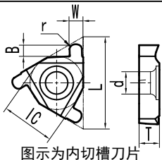
图示为内切槽刀片
