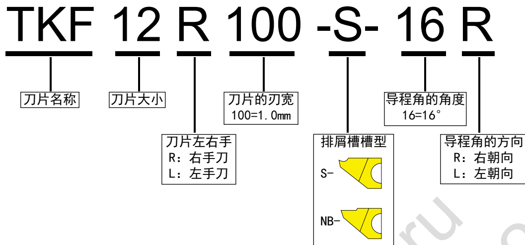
TKF 系列刀片导程角命名示例
