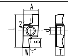
C、D、E 系列刀片式样
